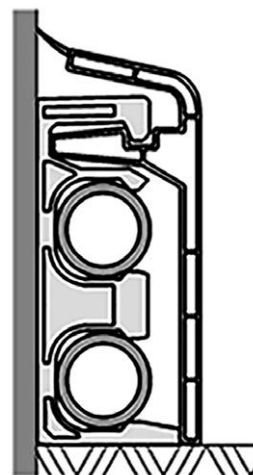
Схема разреза закрытого трубопровода
